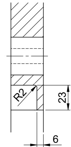
A-A MAßSTAB 1 : 2
