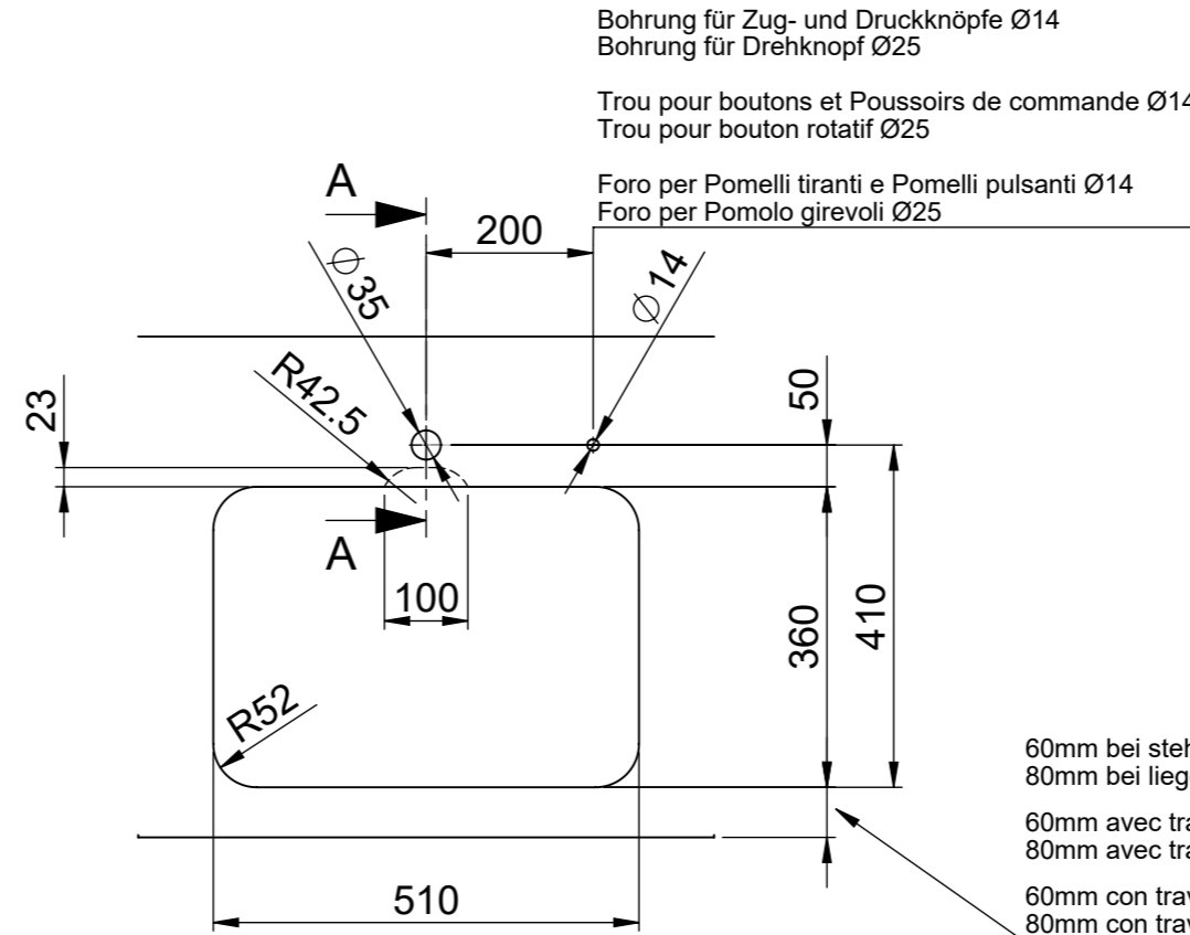
DETAIL X MAßSTAB 1 : 2
