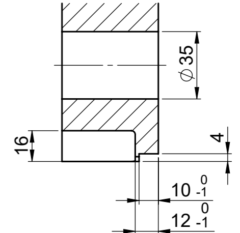
A-A (1 : 2)
