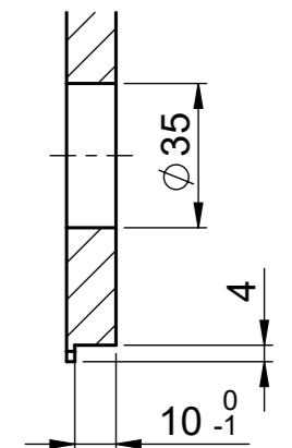
A-A (1 : 2)
