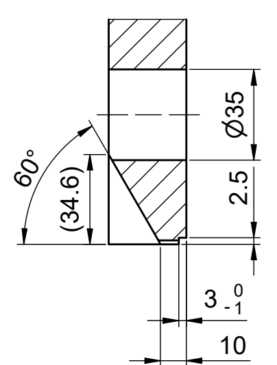
A-A (1 : 2)
