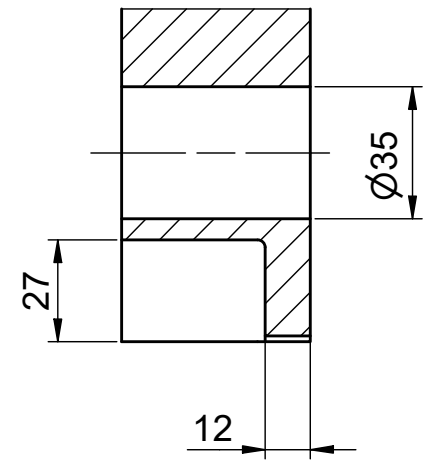
A-A (1:2)
