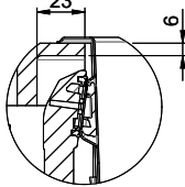
DETAIL Y MAßSTAB 1 : 2
