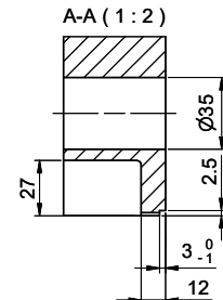
A-A (1 : 2)
