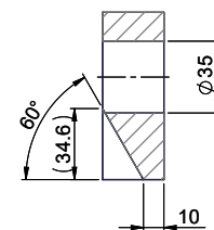
A-A ( 1 : 2 )
