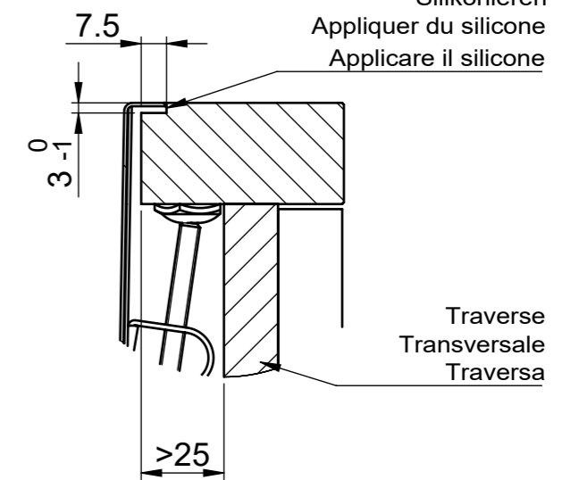
Y (1 : 2)
