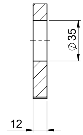
A-A (1 : 2)
