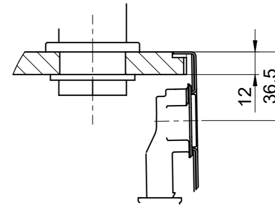
X (1 : 2)
