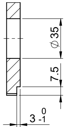
A-A (1 : 2)
