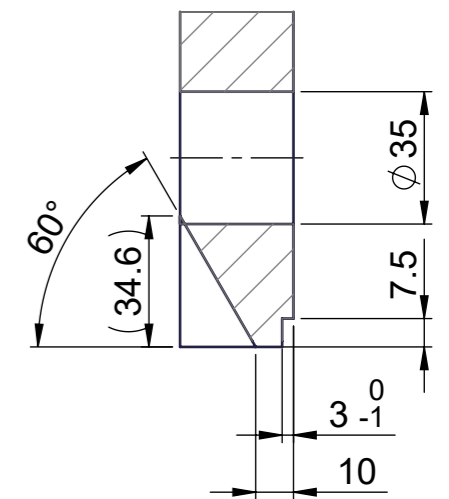
A-A ( 1 : 2 )
