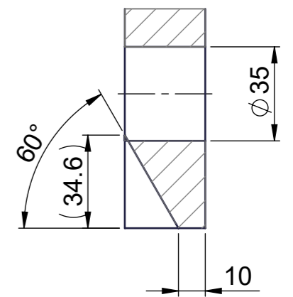
A-A ( 1 : 2 )
