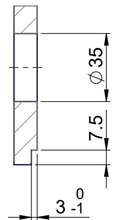
A-A ( 1 : 2 )
