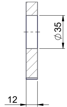
A-A (1 : 2)
