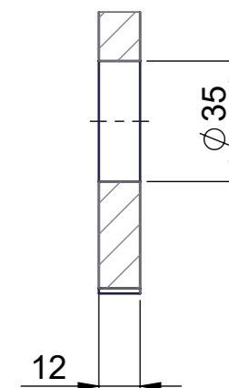
A-A ( 1 : 2 )
