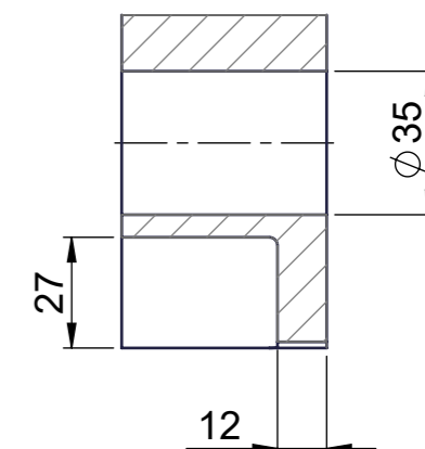
A-A ( 1 : 2 )
