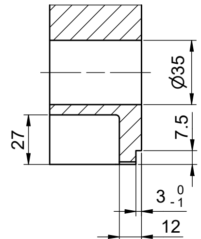
A-A (1:2)
