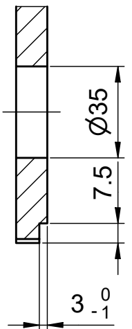
A-A (1:2)
