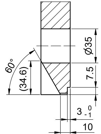
A-A (1:2)
