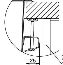
DETAIL Y MAßSTAB 1 : 2
