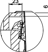
DETAIL Y MASSSTAB 1 : 2
