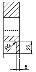
A-A MAßSTAB 1 : 2
