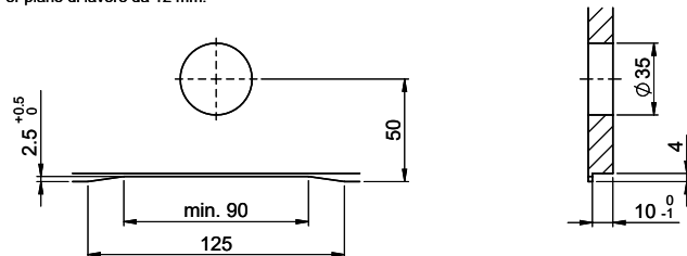
A-A (1 : 2)
