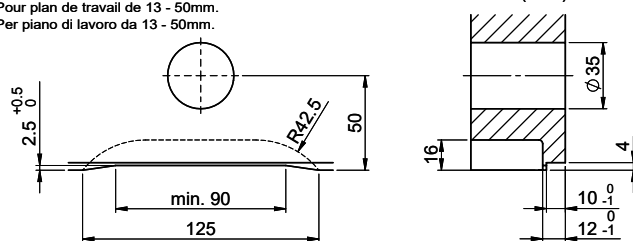
A-A (1 : 2)
