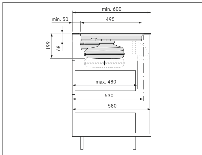
Einbauausschnitt PURA 600 mm / Découpe PURA 600 mm
