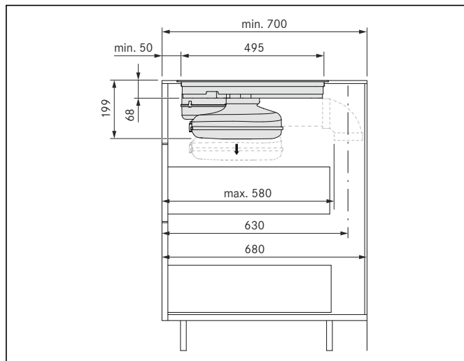
Einbauausschnitt PURA 700 mm / Découpe PURA 700 mm
