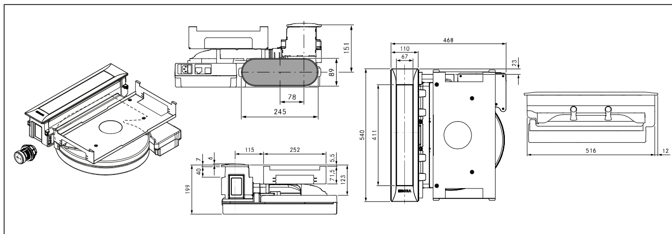
Kochfeldabzugssystem PKAS3/PKAS3AB / Système aspirant de table de cuisson PKAS3/PKAS3AB
