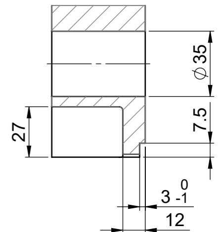
A-A (1 : 2)
