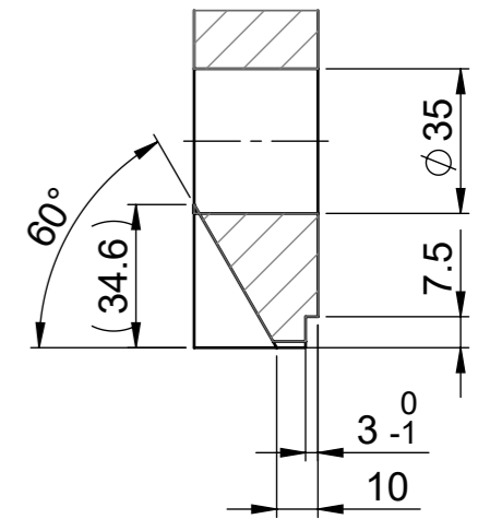
A-A (1 : 2)
