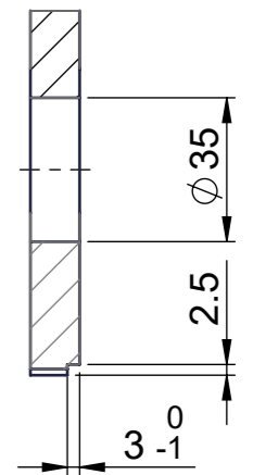
A-A (1 : 2)
