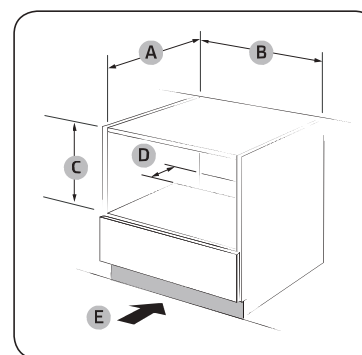
Struttura a incasso sotto lavello (mm)
