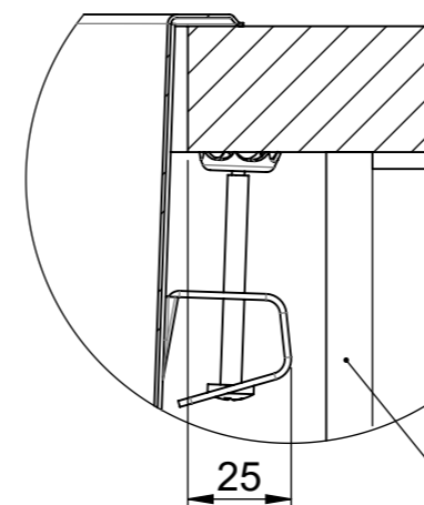
DETAIL Y MAßSTAB 1 : 2
