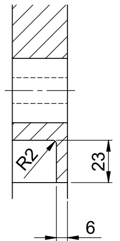
A-A MAßSTAB 1 : 2
