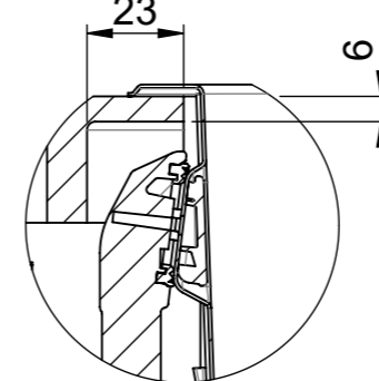
DETAIL X MAßSTAB 1 : 2
