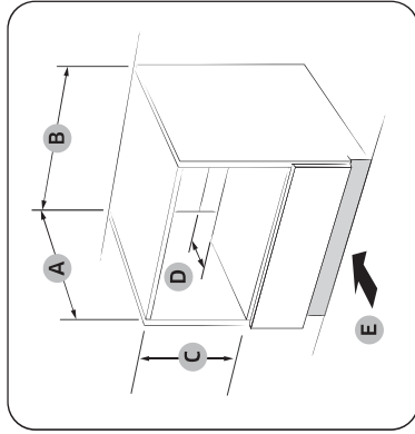
Struttura a incasso sotto lavello (mm)
