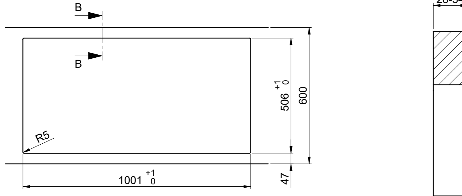
B-B (1 : 2)
