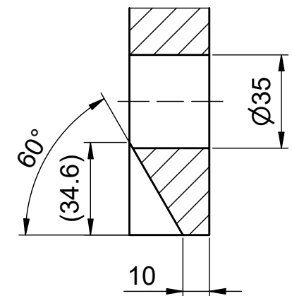
A-A (1:2)
