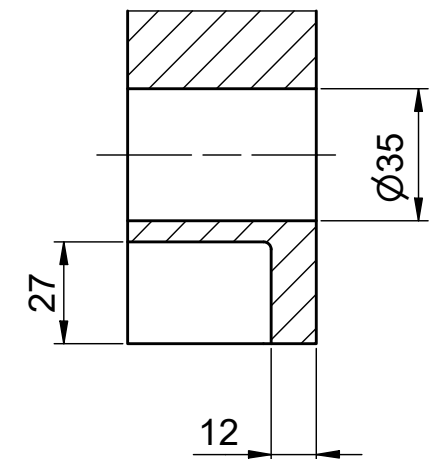
A-A (1:2)
