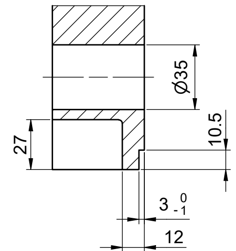
A-A (1:2)
