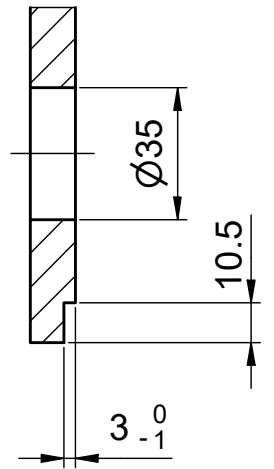
A-A (1:2)
