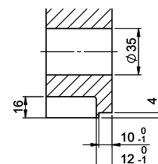
A-A (1 : 2)
