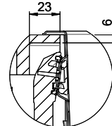
DETAIL Y MAßSTAB 1 : 2
