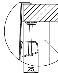
DETAIL Y MAßSTAB 1 : 2
