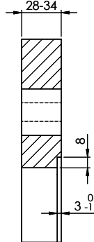
A-A (1 : 2)
