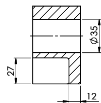
A-A (1 : 2)
