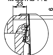
DETAIL Y MAßSTAB 1 : 2
