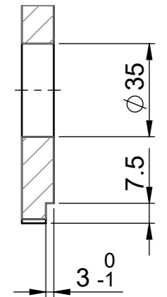
A-A (1 : 2)
