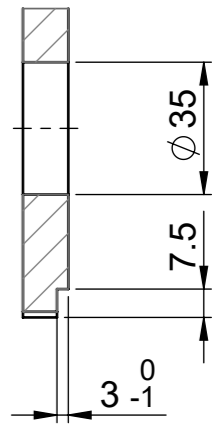
A-A (1 : 2)
