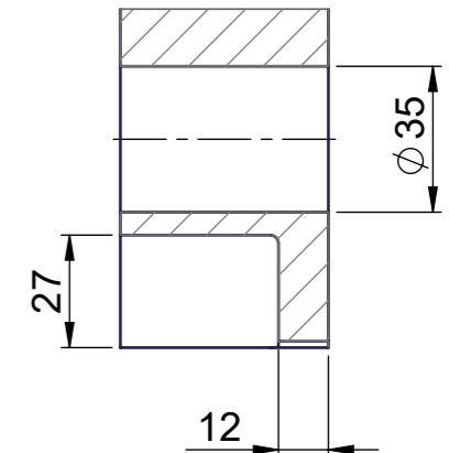
A-A (1 : 2)
