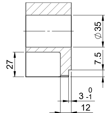
A-A (1 : 2)
