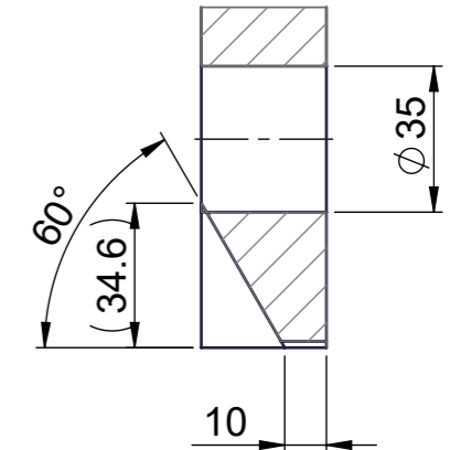
A-A (1 : 2)
