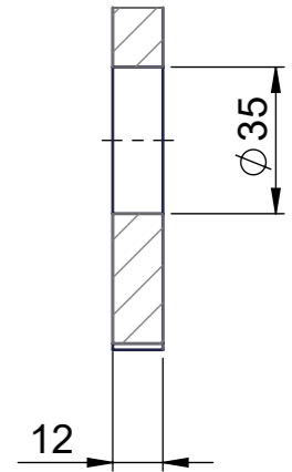
A-A (1 : 2)
