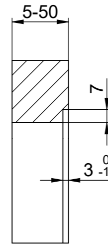
A-A (1 : 2)
