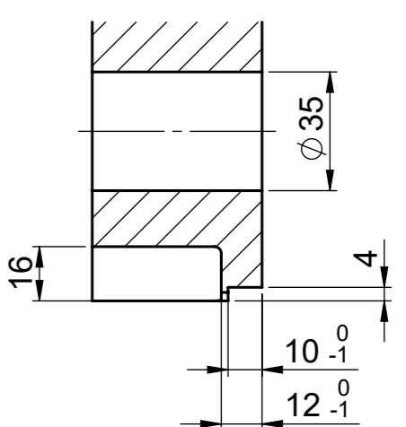
A-A (1 : 2)
