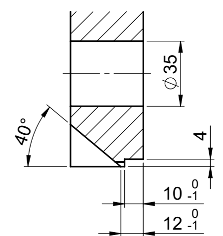
A-A (1 : 2)
