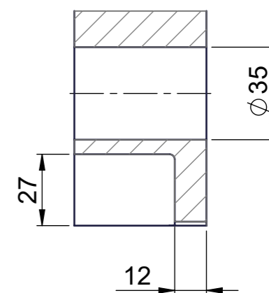
A-A (1 : 2)
