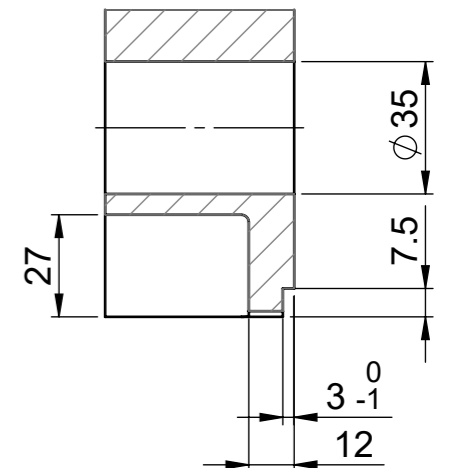
A-A (1 : 2)
