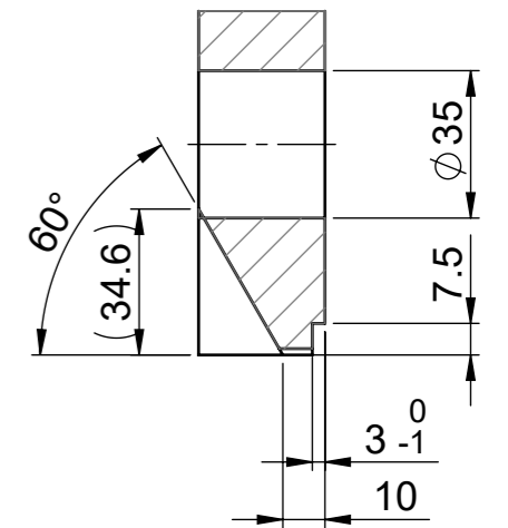
A-A (1 : 2)
