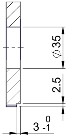
A-A ( 1 : 2 )
