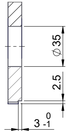
A-A (1 : 2)
