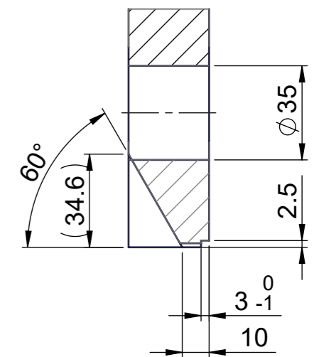
A-A (1 : 2)
