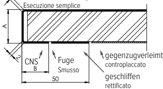
Schnitt A-A / Intaglio A-A Einfache Ausführung Esecuzione semplice
