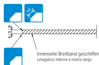
Top Ausführung Esecuzione superiore
