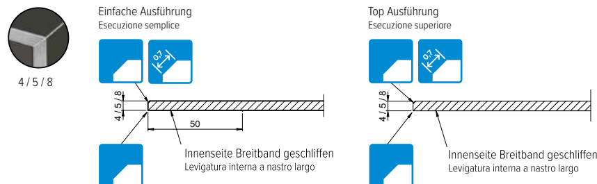
Schnitt A-A / Intaglio A-A
