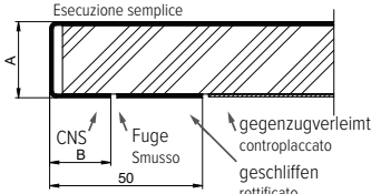
Schnitt A-A / Intaglio A-A Einfache Ausführung Esecuzione semplice
