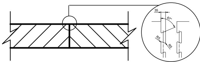
Detail Z: Ausschnitt Crea / Dettaglio Z: intaglio Crea
