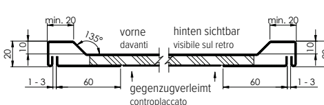
Schnitt A-A / Intaglio A-A
