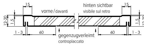
Schnitt A-A / Intaglio A-A
