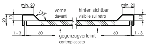
Schnitt A-A / Intaglio A-A
