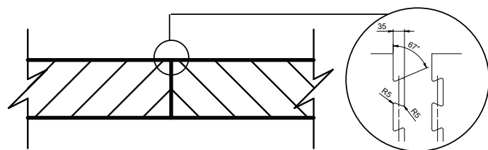
Detail Z: Ausschnitt Crea / Dettaglio Z: intaglio Crea
