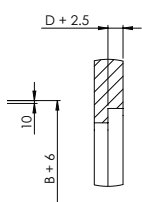
Schnitt A-A / Intaglio A-A
