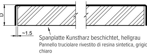
Schnitt A-A / Intaglio A-A
