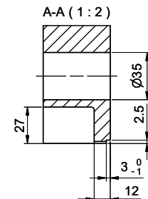
A-A (1 : 2)
