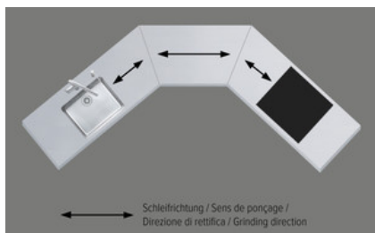
Modell Offener U-Winkel
